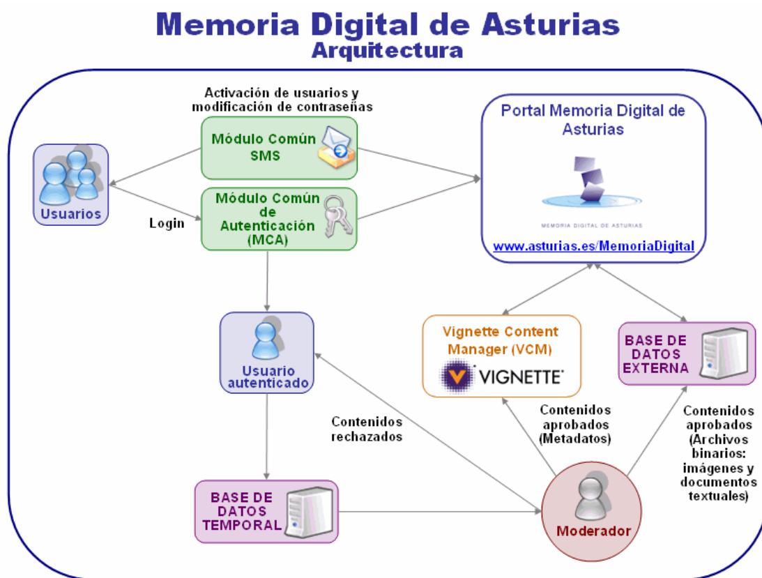
Ilustración I. Arquitectura de la Memoria Digital de Asturias
