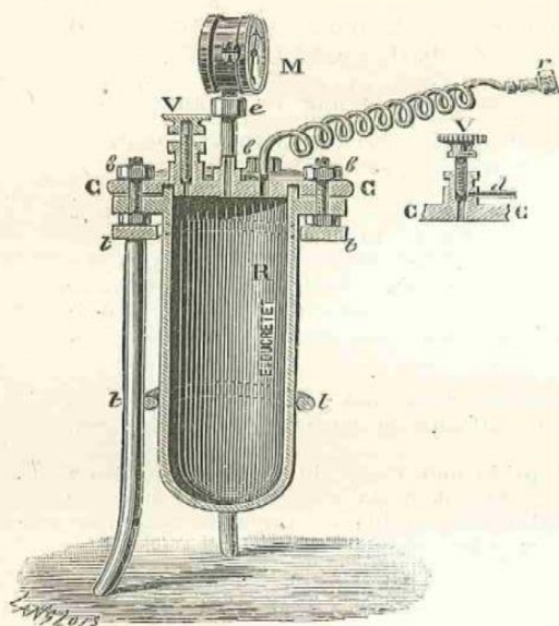
Fig. 351. — Stérilisateur de M. d'ARSONVAL par simple pression de \text{CO}_2 .
