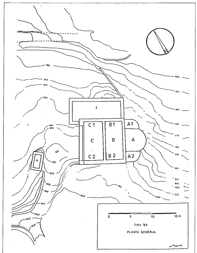
Fig. 1.—Organización en sectores de la superficie de la iglesia
