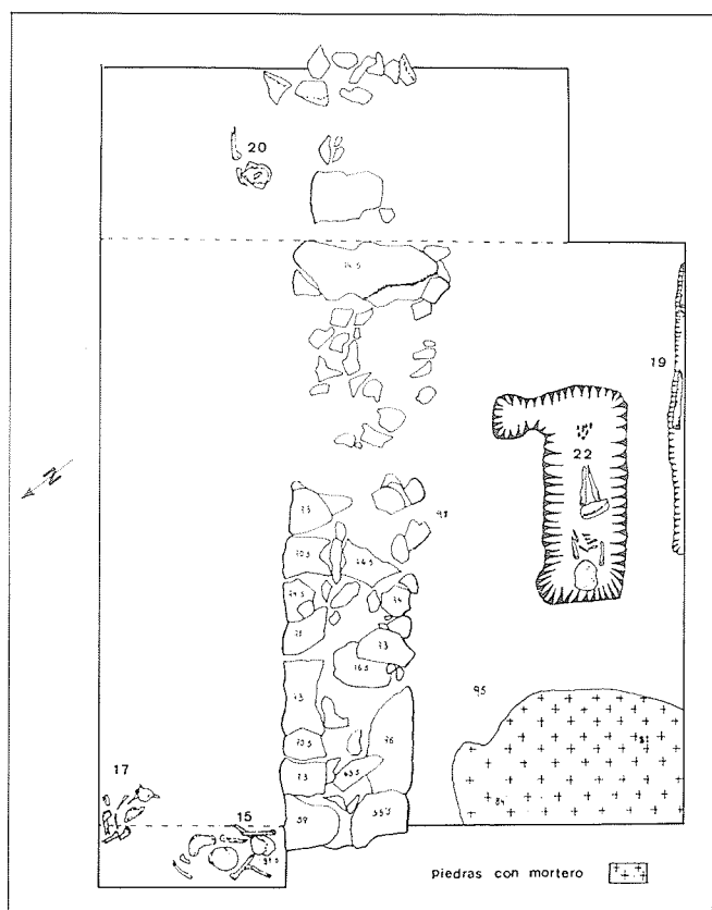
Fig. 5.—CATA C-1. TINA-86.
