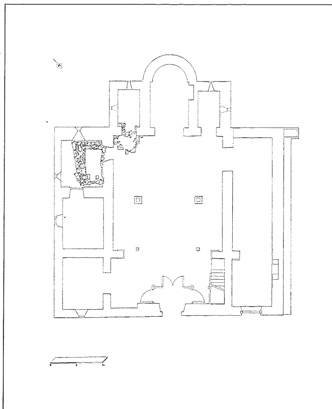
Fig. 2.—Restos conservados de la planta de la Iglesia del siglo X.
