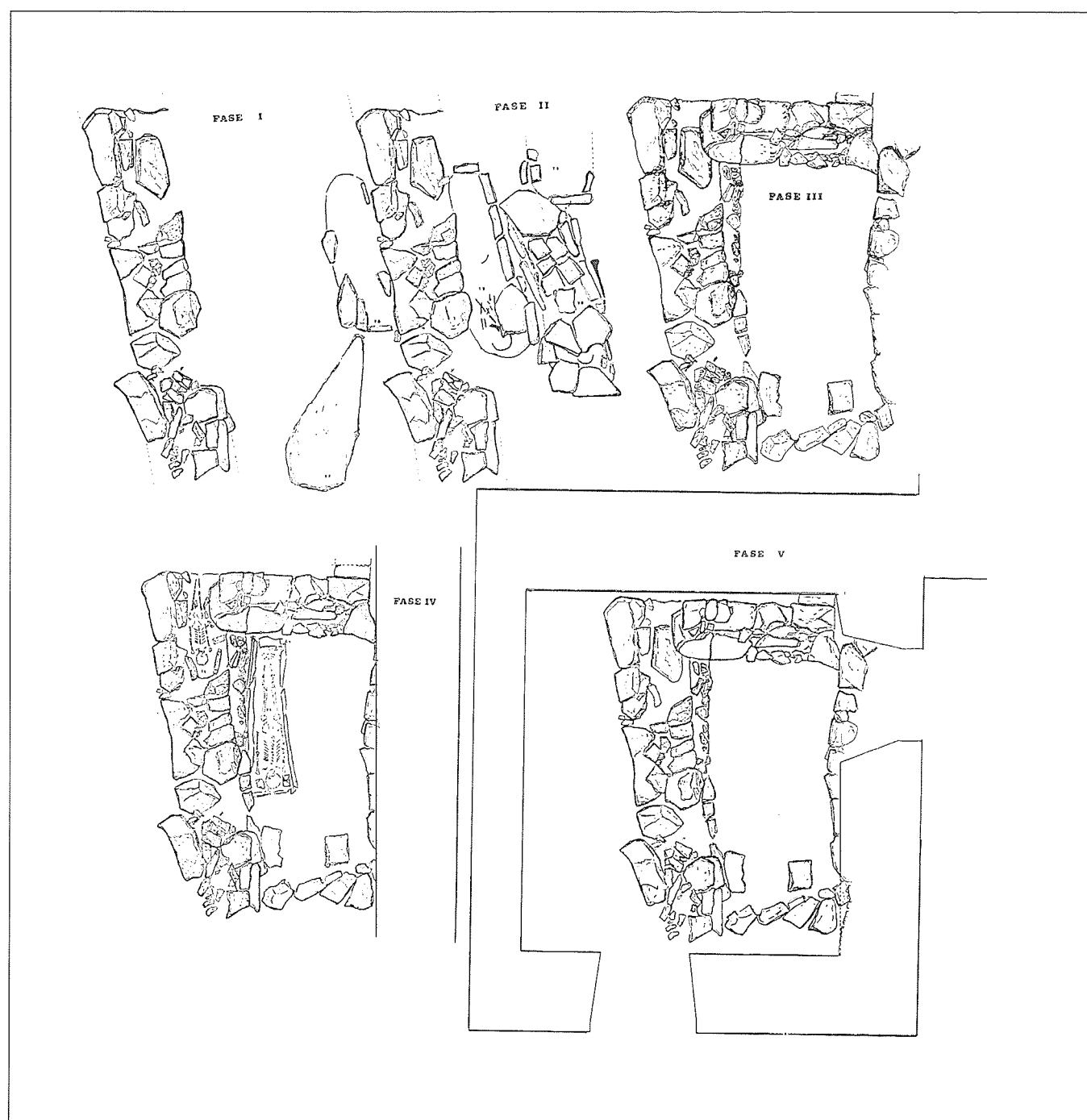
Fig. 1.—Fases constructivas de la Iglesia de San Vicente de Serrapio.
