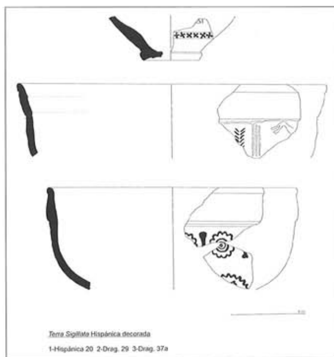
Figura 3.—Formas decoradas de Terra Sigillata Hispanica de los siglos I y II d.C. (Dibujo: J. Mon).
