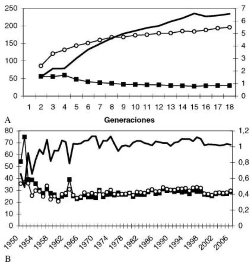
Figura 2. Evolución del \bar{N}_e realizado ( \bar{N}_e , cuadrados negros, eje izdo.), tamaño efectivo por coascendencias ( \bar{N}_{ec} , círculos blancos, eje izdo.) y medida de subdivisión ( S , línea continua gruesa, eje dcho.) en la población de ratones (A) y en la población de toro de lidia (B).
